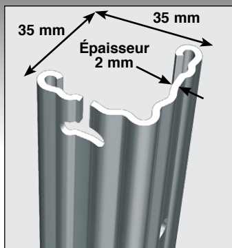
Vue de la section Cortech 35
